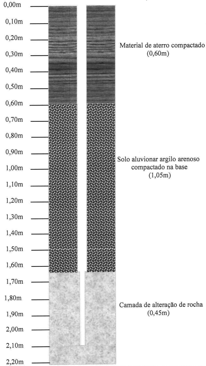
Fig. 01: Perfil esquemático em SP 01 com profundidade de 2,10m.
