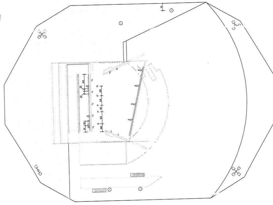
PLANTA BAIXA PONTOS ELÉTRICOS Esc. 1/10
