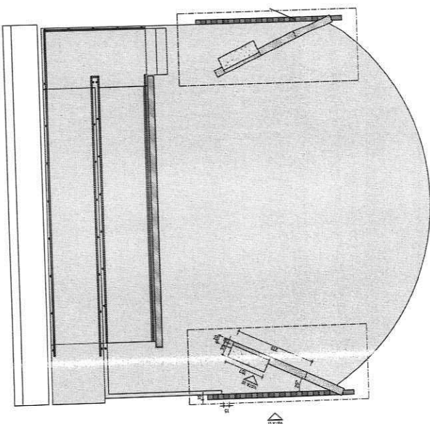
LOCALIZAÇÃO DO QUADRO E PAINEL METÁLICOS
