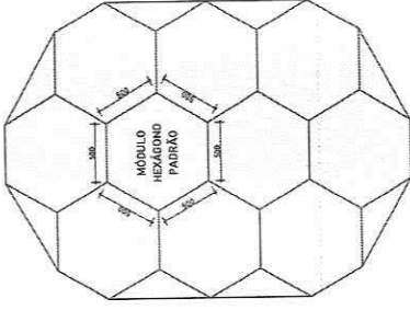
COMPOSIÇÃO DO MÓDULO CONFORME A MALHA HEXAGONAL DEFINIDA Esc. 1:200
